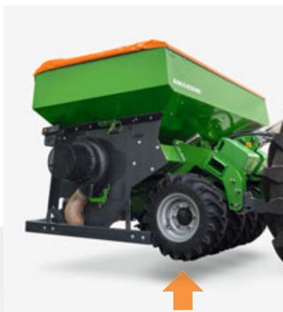
FTender с фронтальным шинным пакером T-Pack F в транспортном положении
