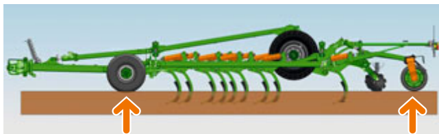
Ведение по глубине за счет опорных колес и катка
