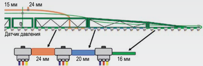
Циркуляция высокого давления DUS pro с конической напорной магистралью на примере AmaSwitch
